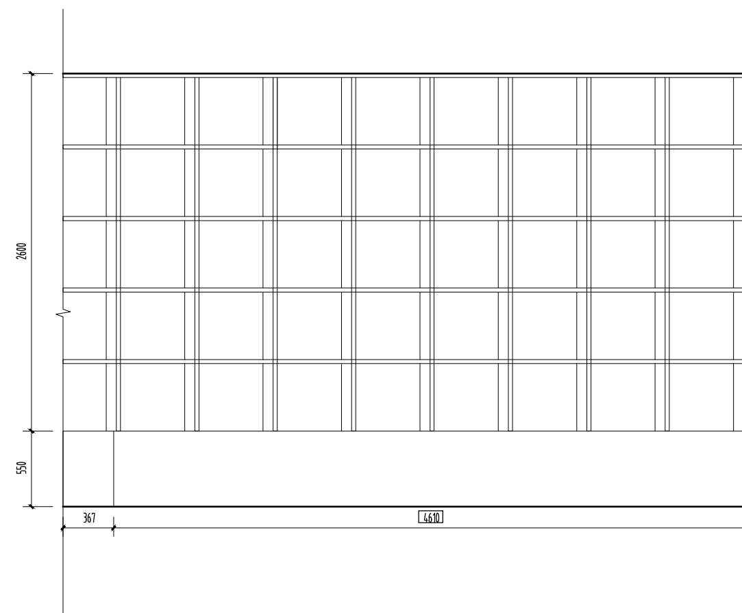
书架 A立面图 1:25
