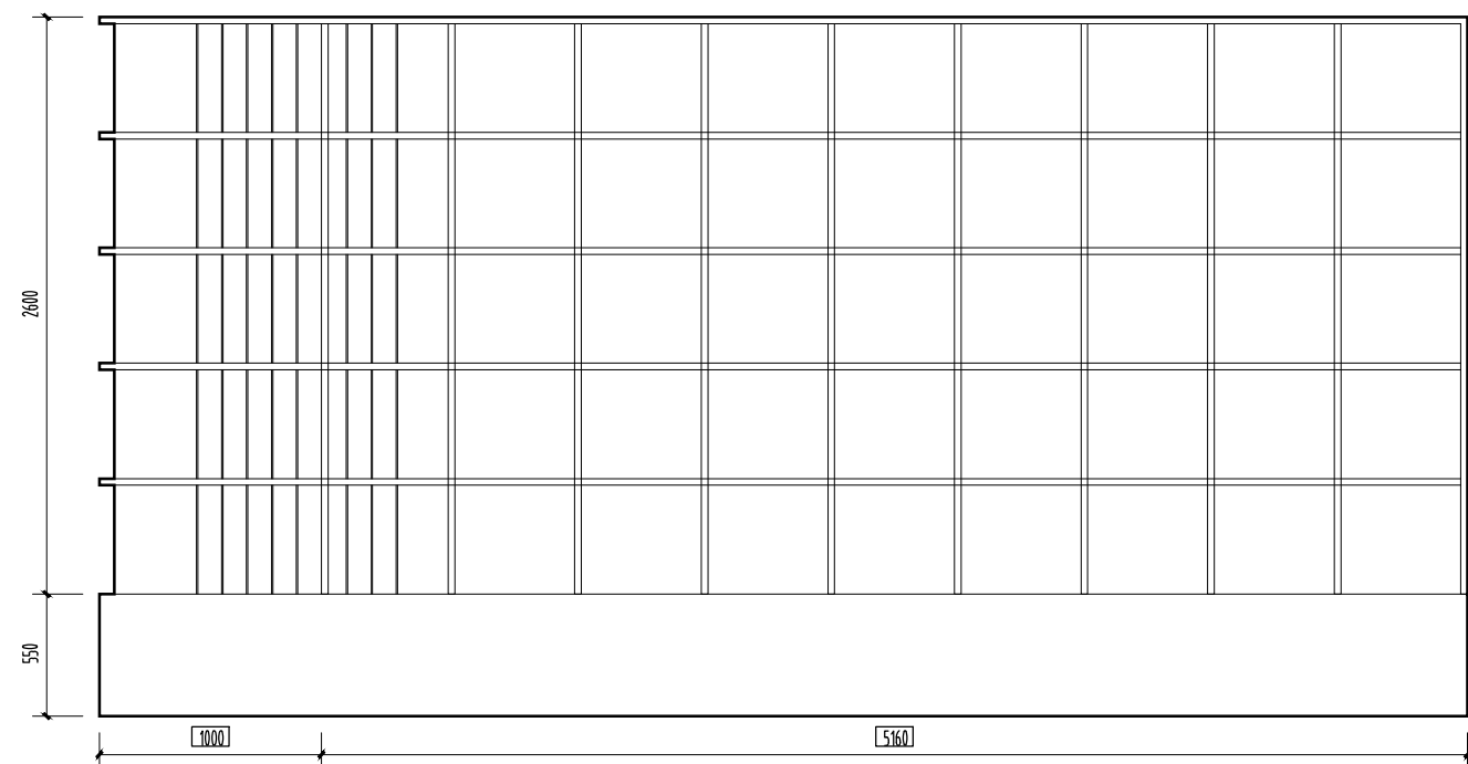
书架 B立面图 1:25
